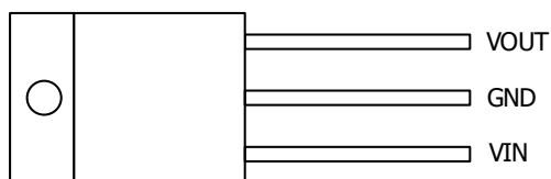
TO220-3L
