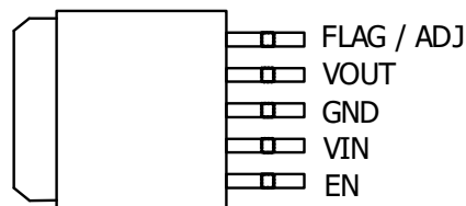
TO263-5L
